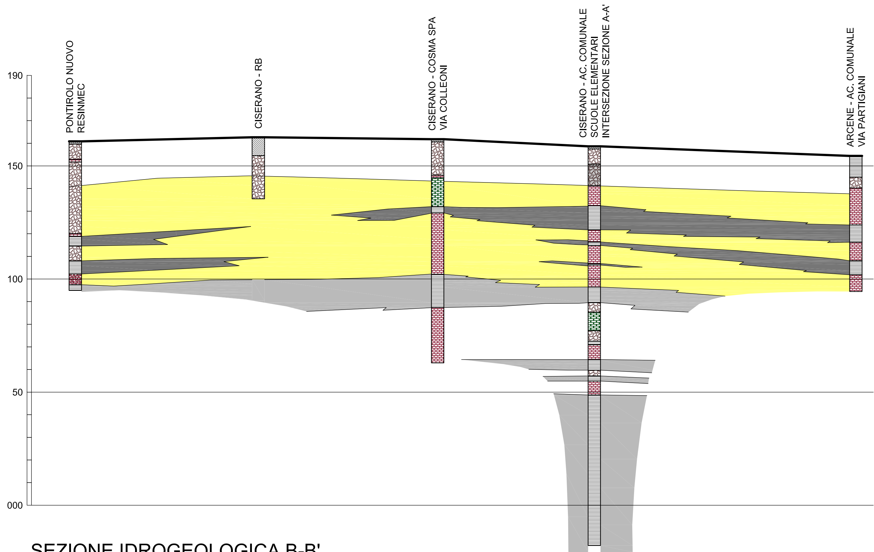
SEZIONE IDROGEOLOGICA B-B'
